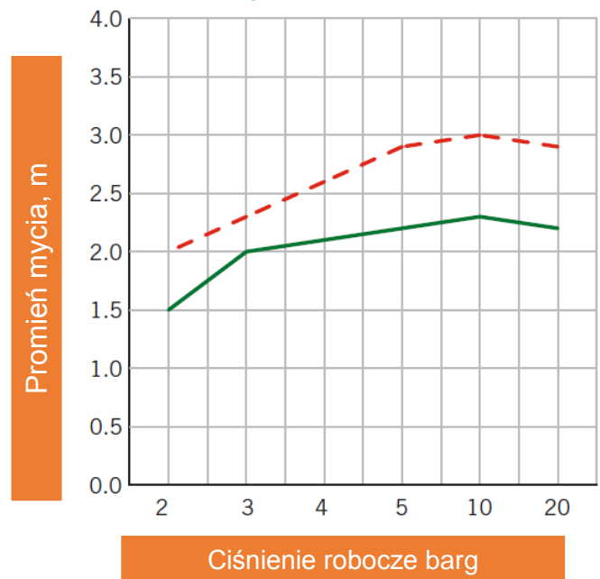
Promień mycia/ Promień zwilżania
