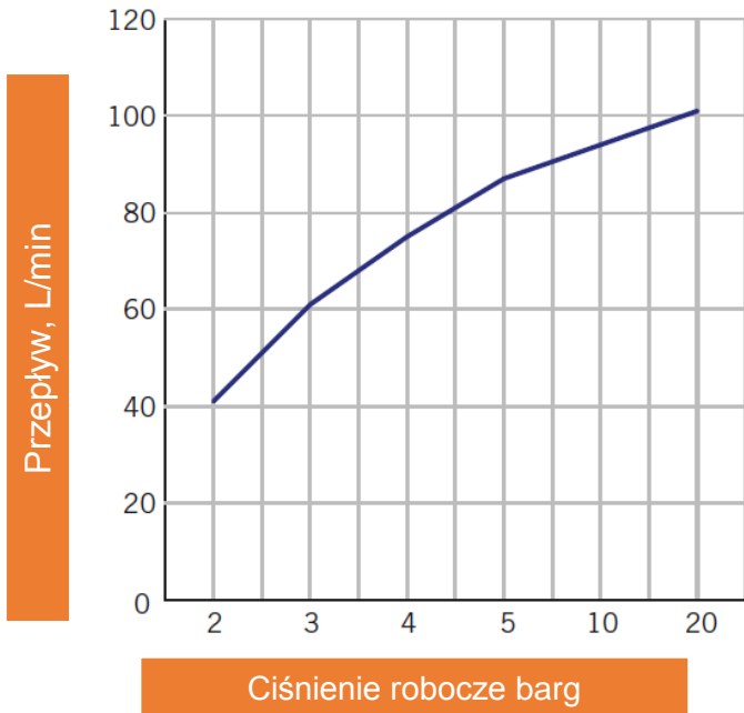
Przepływ w zależności od ciśnienia
